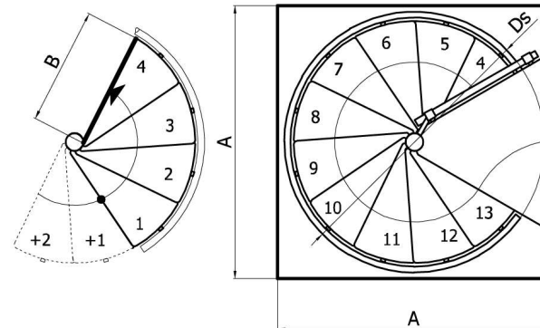
Půdorys
