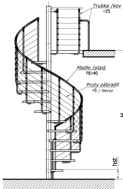
Pohled z boku
